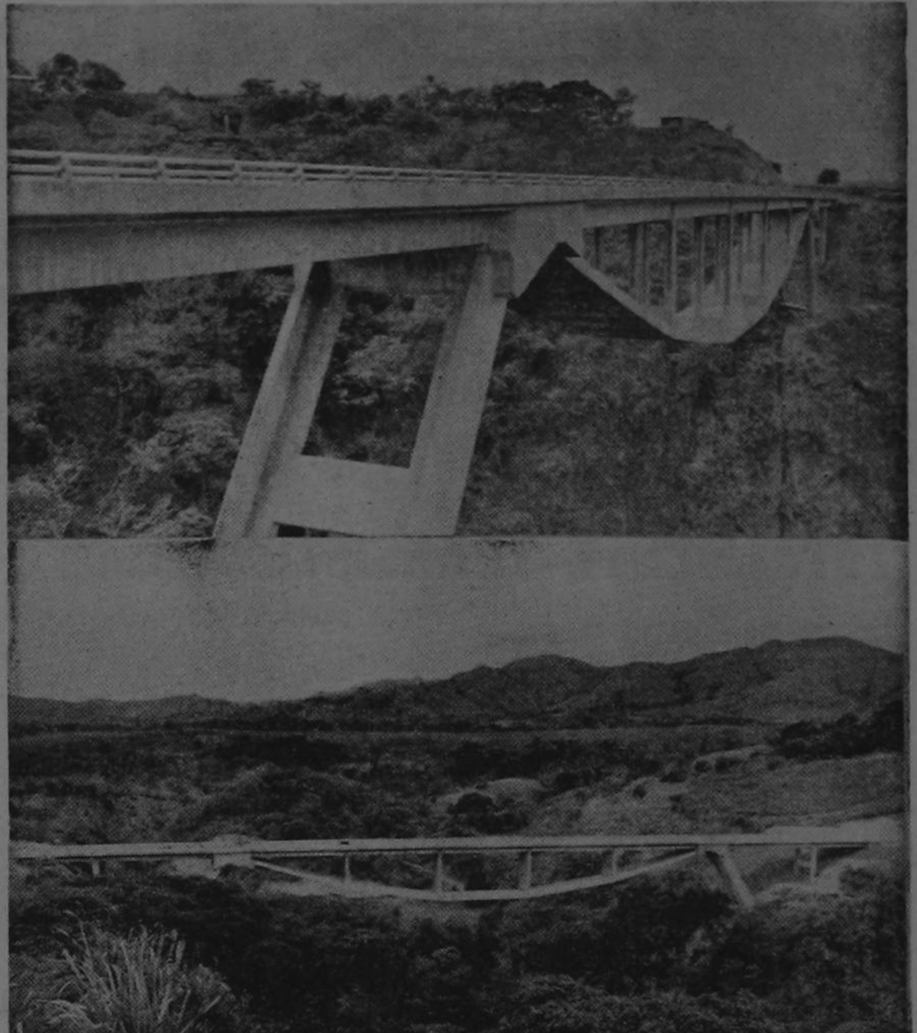
Puente sobre el Río Colorado. Longitud, 207 metros. Costo, casi 8 millones de colones. El diseño fue hecho por las firmas Indeca y T. Y. Lin. Construido por la empresa Carrez International. Por su estilo colgante es único en su género y el más notable de todos los puentes de Costa Rica.
